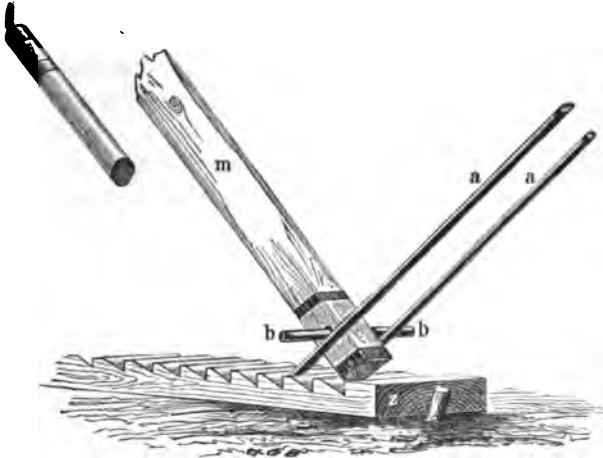
Fig. 140.—Wohmann's machine,
